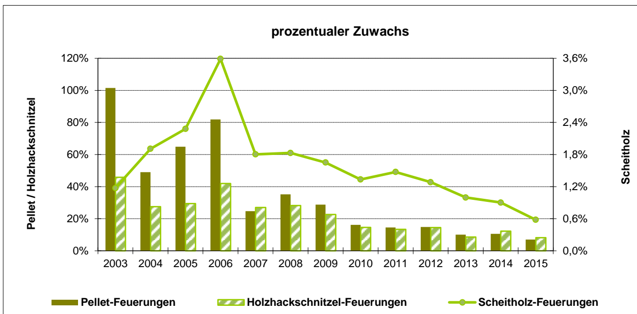
Abb. 3: Prozentualer Zuwachs bei Holzfeuerungen < 1 MW in Niedersachsen
