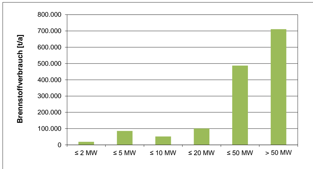
Abb. 11: Brennstoffverbrauch der Holzfeuerungsanlagen > 1 MW nach Größenklassen
