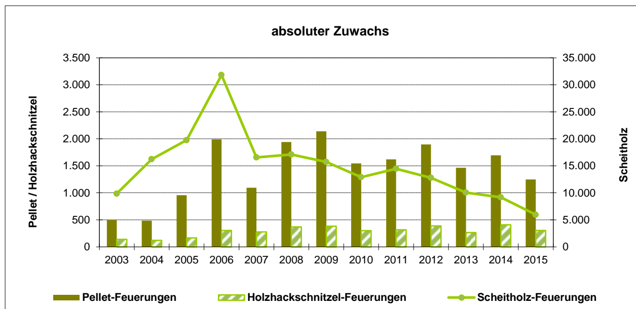
Abb. 1: Absoluter Zuwachs bei Holzfeuerungen < 1 MW in Niedersachsen
