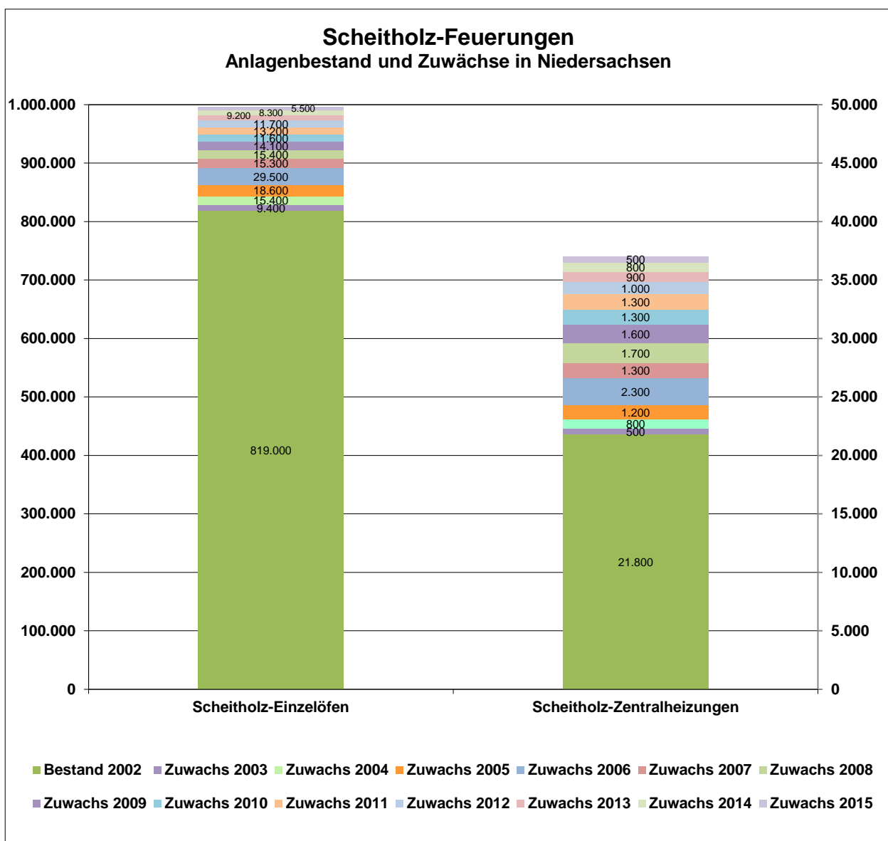
Abb. 4: Scheitholz-Feuerungen – Entwicklung des Bestandes nach Anlagenkategorien
