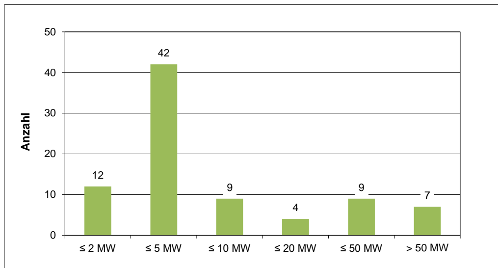
Abb. 7: Größenverteilung der Holzfeuerungsanlagen > 1 MW
