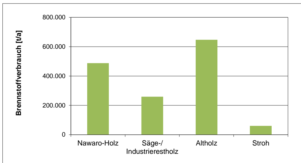
Abb. 12: Verteilung der eingesetzten Brennstoffe in Holzfeuerungsanlagen > 1 MW
