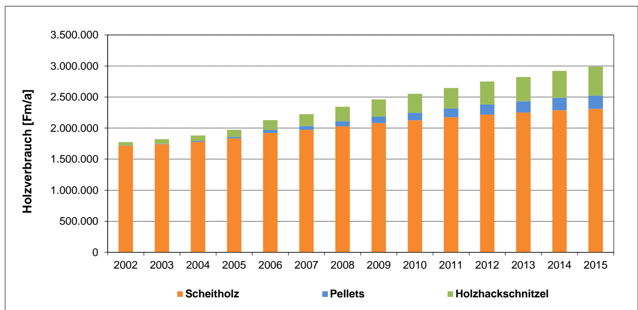
Abb. 9: Holzverbrauch der Feuerungen < 1 MW in Niedersachsen
