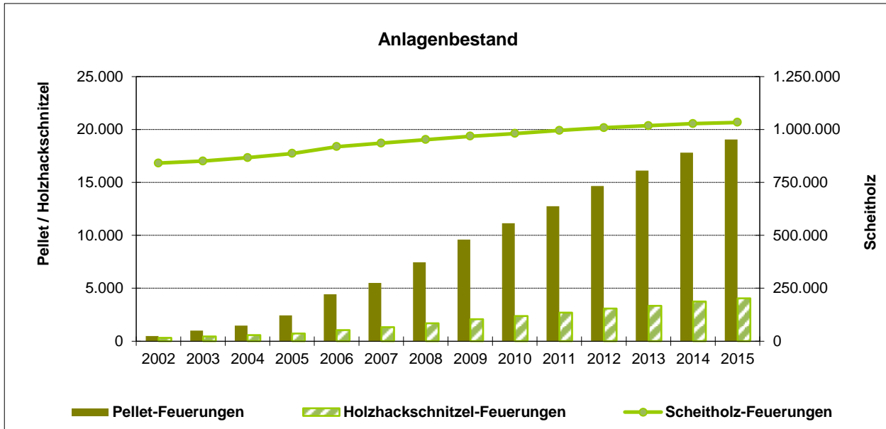
Abb. 2: Anlagenbestand an Holzfeuerungen < 1 MW in Niedersachsen
