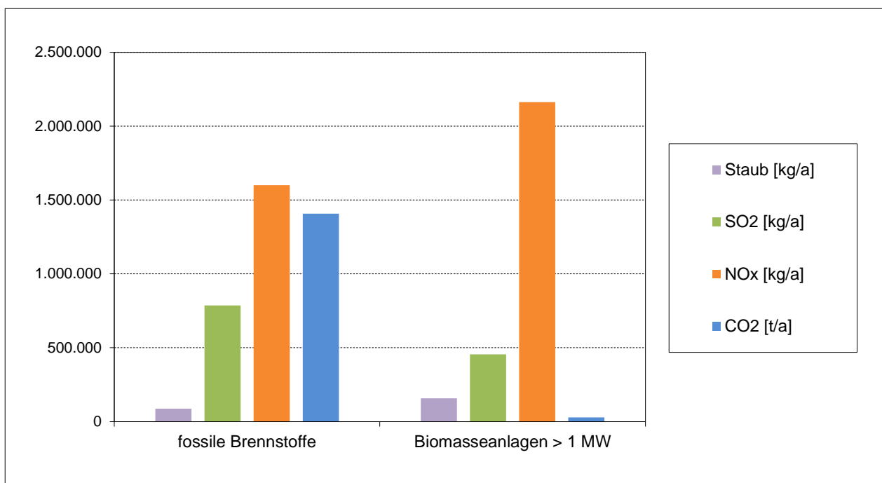
Abb. 15: Emissionsvergleich zwischen Holzfeuerungsanlagen > 1 MW und fossil befeuerten Anlagen
