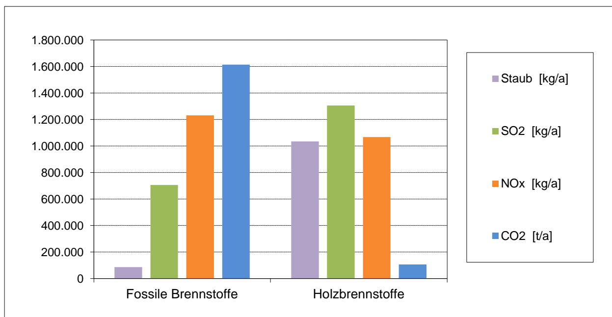
Abb. 14: Emissionsvergleich zwischen Holzfeuerungen und fossil befeuerten Heizanlagen < 1 MW
