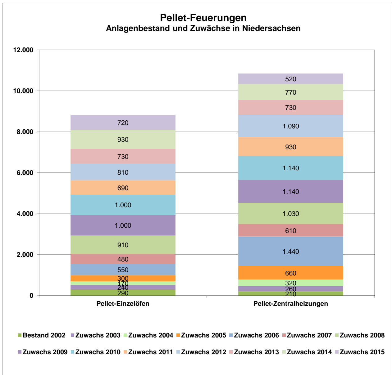
Abb. 5: Pellet-Feuerungen – Entwicklung des Bestandes nach Anlagenkategorien
