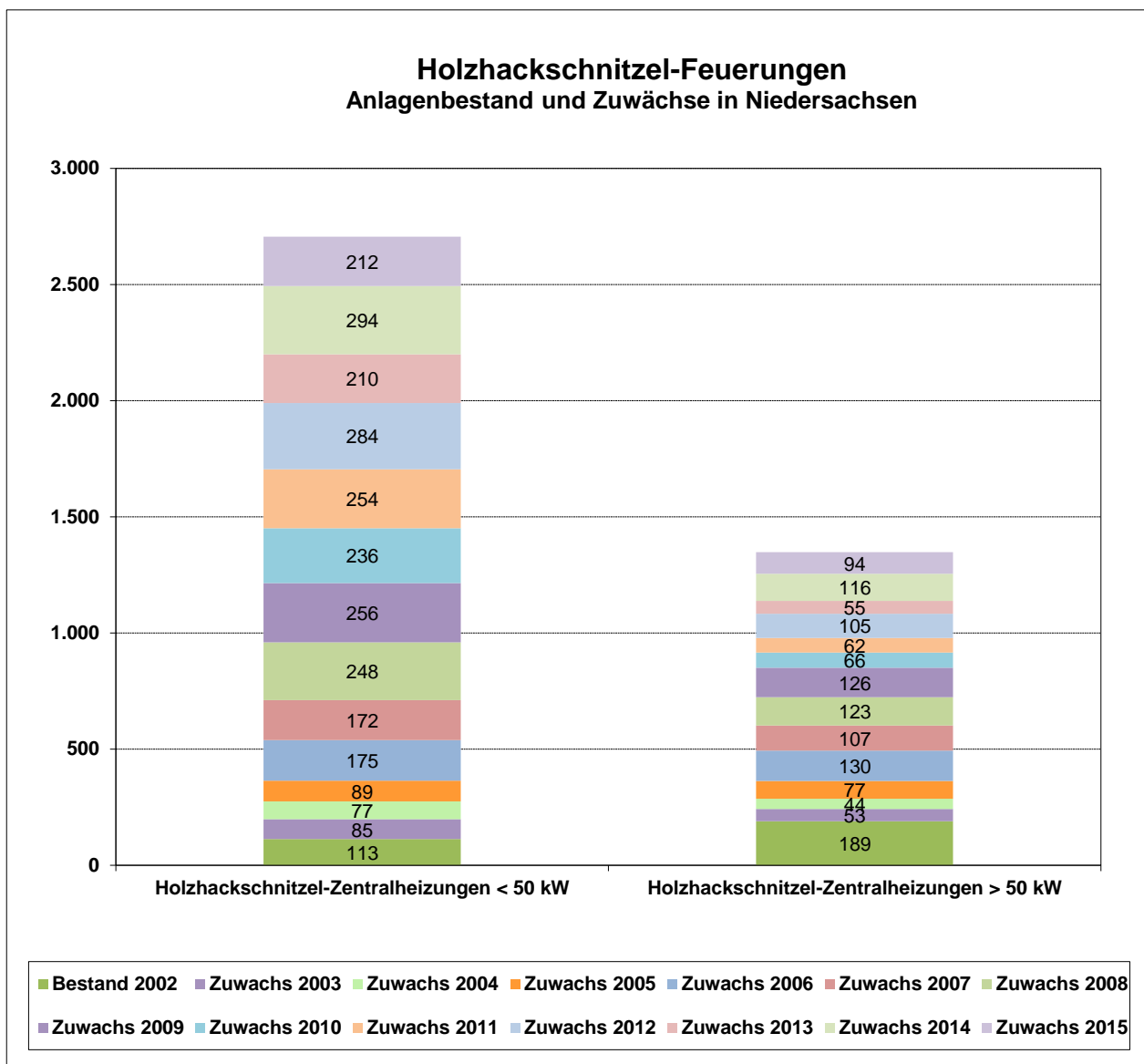
Abb. 6: Holzhackschnitzel-Feuerungen – Entwicklung des Bestandes nach Anlagenkategorien
