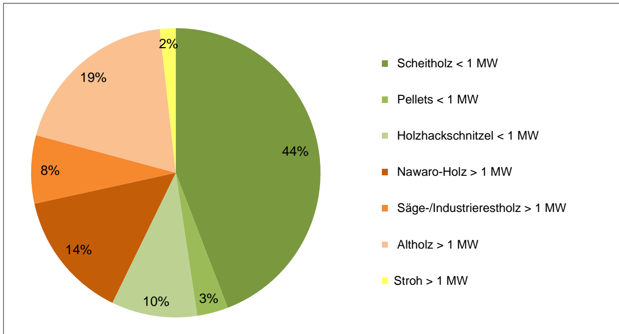
Abb. 13: Gesamtverteilung aller eingesetzten Brennstoffe
